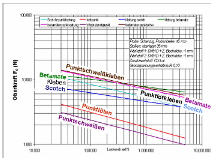
Schwingfestigkeiten der konkurrierenden Prozesse
